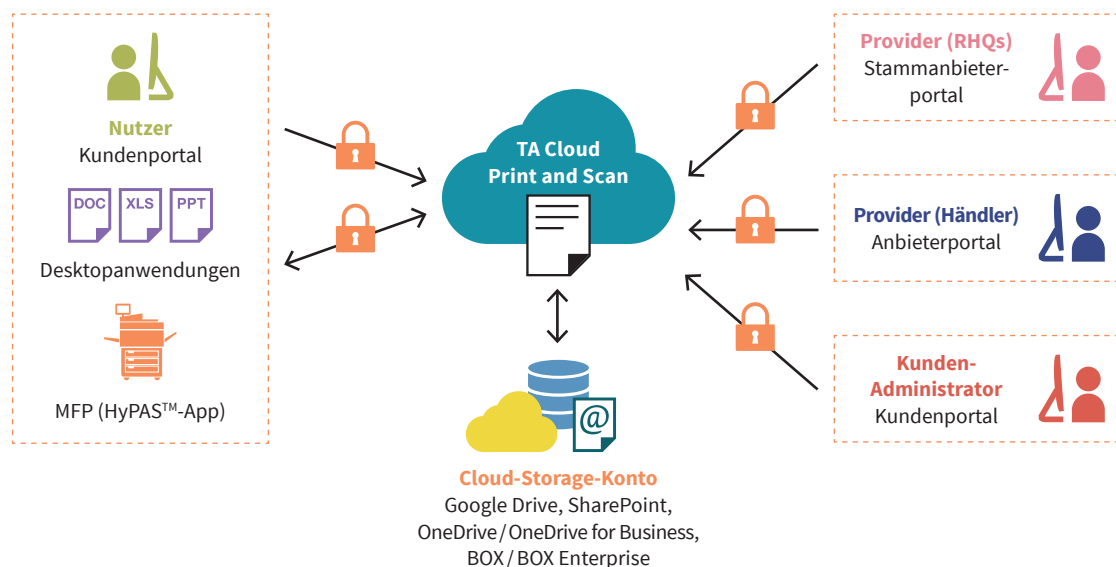
(Abb. 1-1) TACPS-Komponenten
